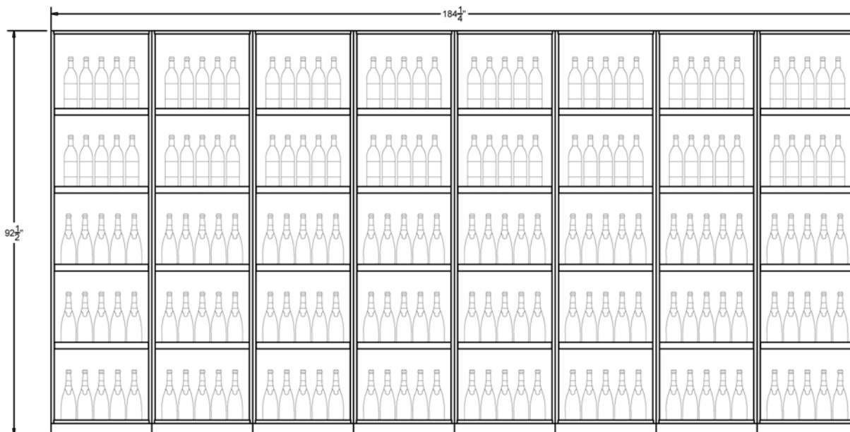
ELEVATION -D-
