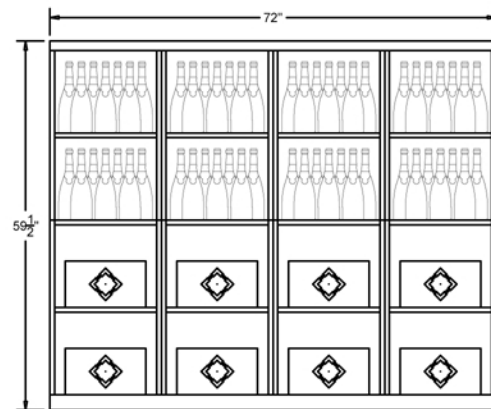
ELEVATION -C- (2X)
