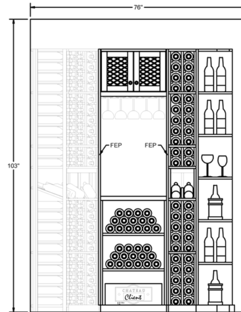
ELEVATION -C-
